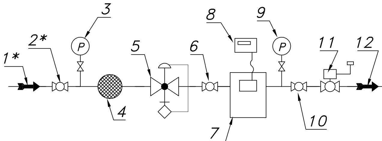
Schemat technologiczny
